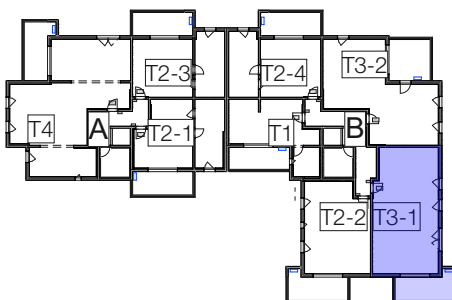
PLAN DU 2ÈME ÉTAGE
