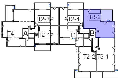
PLAN DU 4ÈME ÉTAGE
